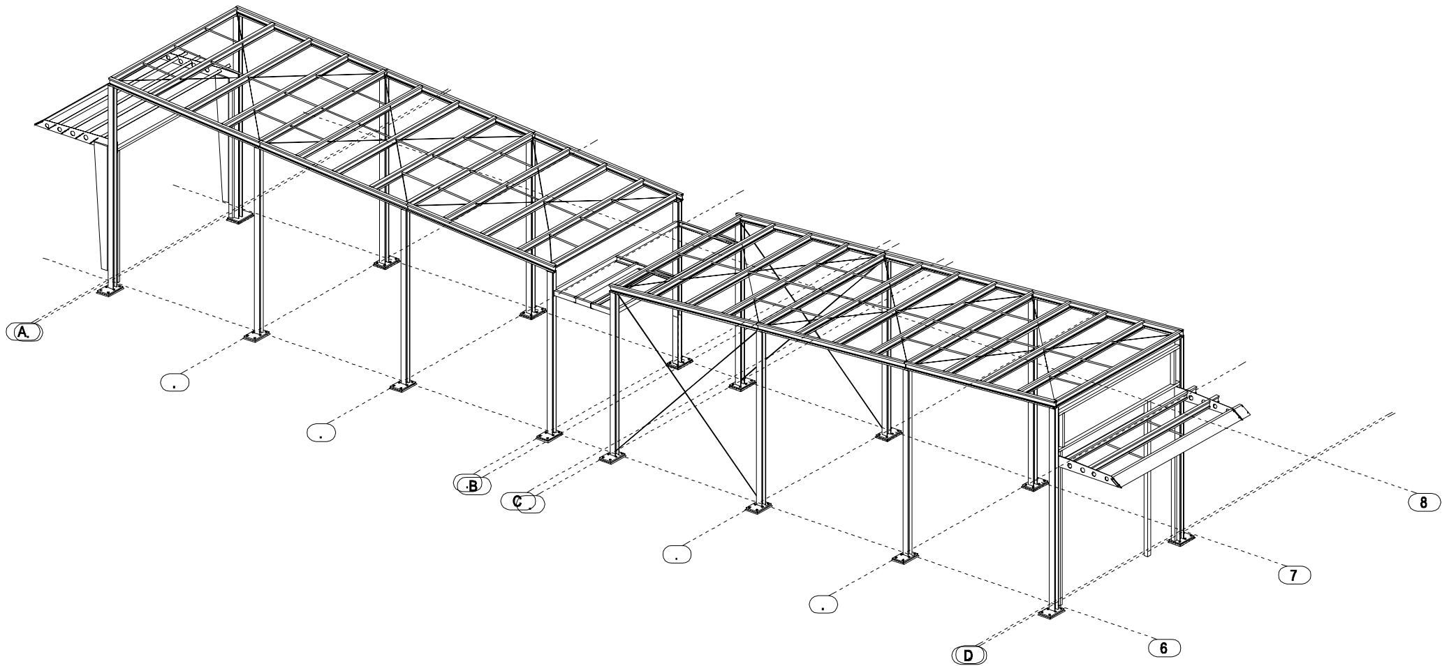
AXONOMETRIA NAVRHOVANEJ OCEĽOVEJ KONŠTRUKCIE
